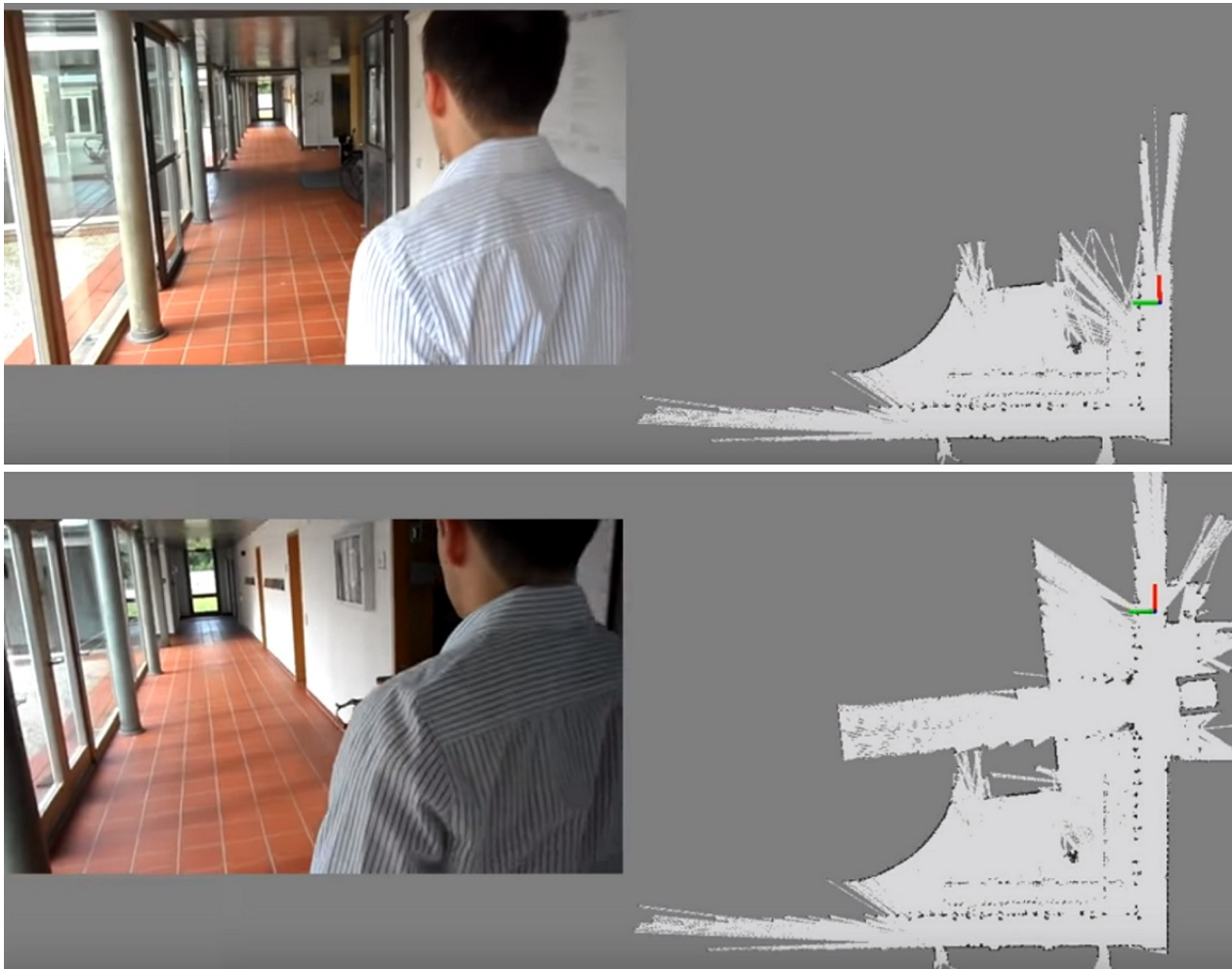
Hector SLAM效果
