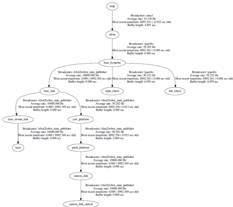
TF树
