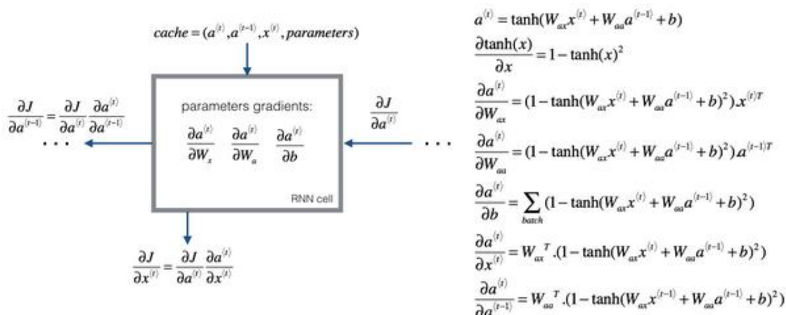
RNN 反向传播示意图：
