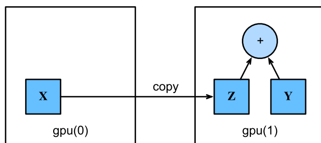
图4.6.1: 复制数据以在同一设备上执行操作。
