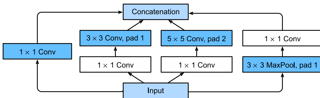
图6.4.1: Inception块的结构。
